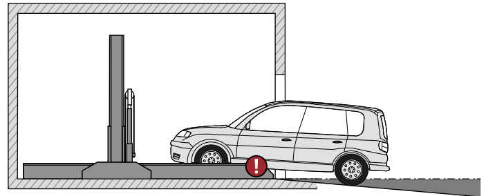
max. 14% gradient
