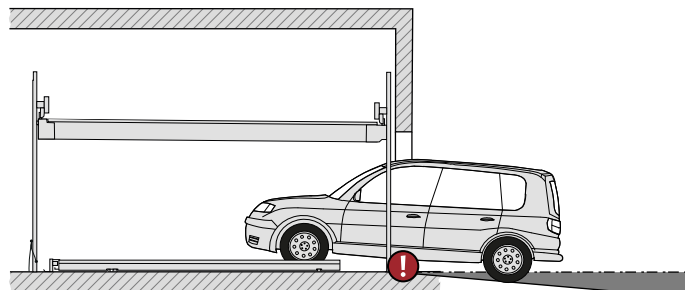
max. 5% gradient
